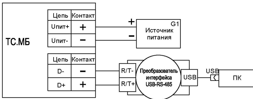
Рисунок 2.17 – Схема измерений выходного сигнала ТС.МБ с помощью источника питания постоянного тока, преобразователя интерфейса USB-RS-485 и ПК
