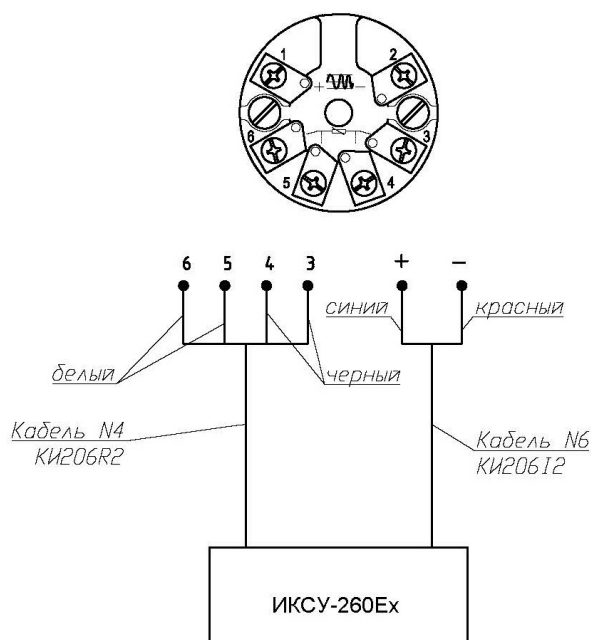
Схема подключения ИП.ХТ-PR, ИП.ХТ-Y к ИКСУ-260Ех в режиме «Симуляция»
