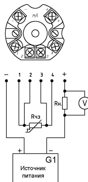
Схема подключения ИП.ХТ-W к магазину сопротивлений R_{чз} , имитирующему сопротивление ЧЭ, источнику питания G1 , сопротивлению нагрузки R_n и вольтметру V
