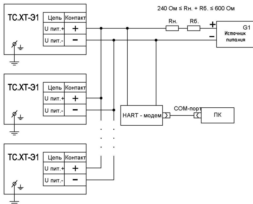
Рисунок Ж.16 – Схема подключения ТС.ХТ-Э1 к сопротивлению нагрузки R н ., сопротивлению R б ., источнику питания G1, HART-модему и ПК в многоточечном режиме
