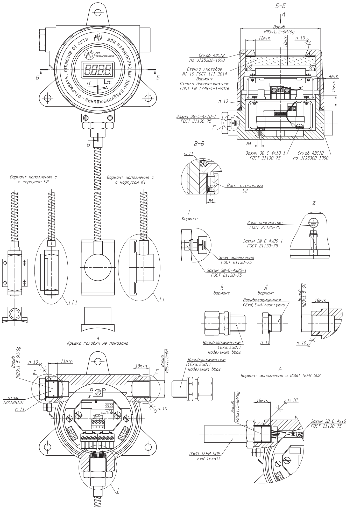
Рисунок 1.8 - Чертеж средств взрывозащиты ТСМУ 011, ТСПУ 011 с головкой типа «Г7/2»
