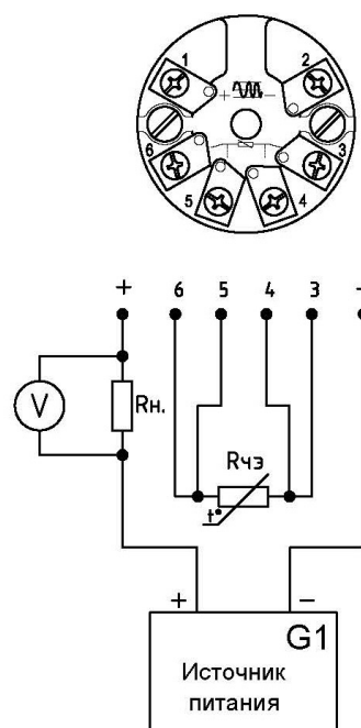
Схема подключения ИП.ХТ-PR, ИП.ХТ-Y к магазину сопротивлений R_{чз} , имитирующему сопротивление ЧЭ, источнику питания G1 , сопротивлению нагрузки R_n и вольтметру V
