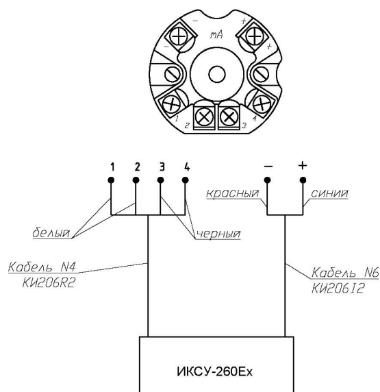
Схема подключения ИП.ХТ-W к ИКСУ-260Ех в режиме «Симуляция»
