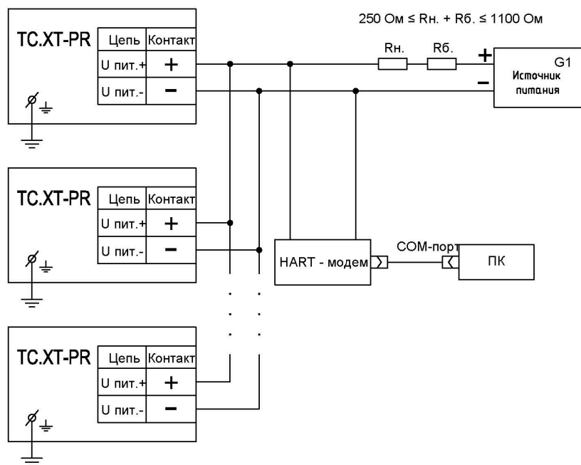
Рисунок К.5 – Схема подключения ТС.XT к сопротивлению нагрузки Rн., сопротивлению Rб., источнику питания G1, HART-модему и ПК в многоточечном режиме
