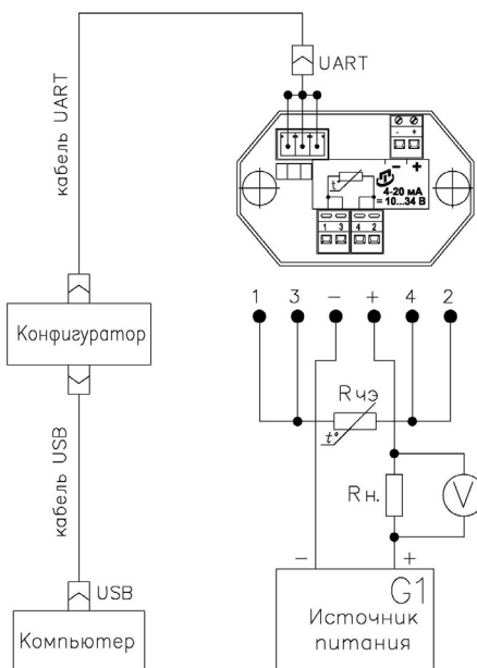
Рисунок Р.1 – Схема подключения ИП, ИП.МП к магазину сопротивлений R_{чэ} , имитирующему сопротивление ЧЭ , источнику питания G1 , сопротивлению нагрузки R_n , вольтметру V , USB-UART-конфигуратору и ПК
