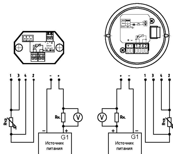
Схема подключения ИП, ИП.ИНД, ИП.МП, ИП.МП.ИНД к магазину сопротивлений R_{чэ} , имитирующему сопротивление ЧЭ, источнику питания G1, сопротивлению нагрузки R_n и вольтметру V
