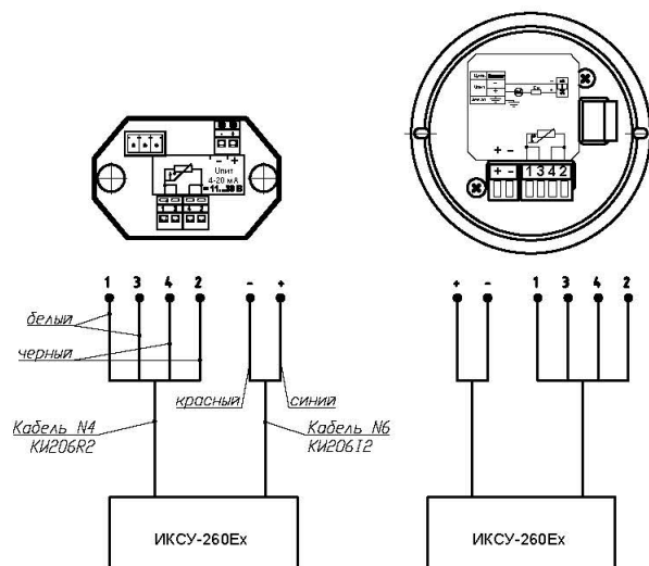
Схема подключения ИП, ИП.ИНД, ИП.МП, ИП.МП.ИНД к ИКСУ-260Ех в режиме «Симуляция»
